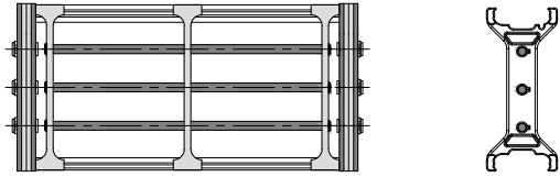
Yatay Separatör Uygulaması Horizontal Separator Application
