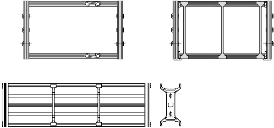
Yatay Separatör Uygulaması Horizontal Separator Application
