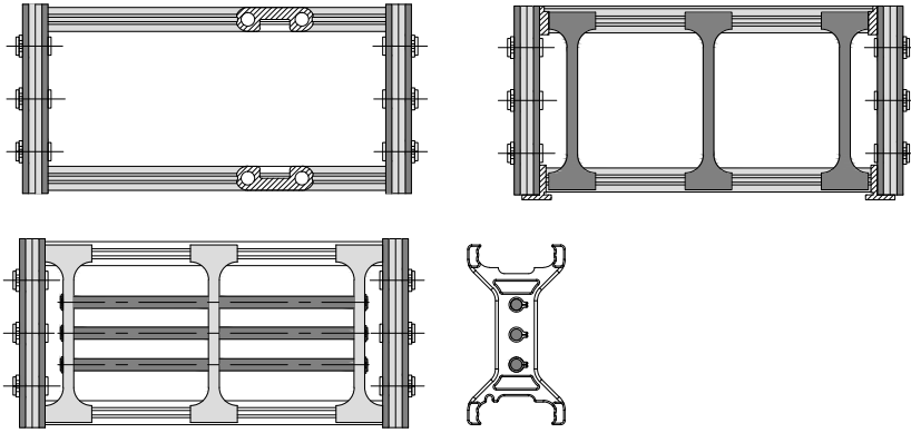
Yatay Separatör Uygulaması Horizontal Separator Application
