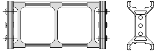
Plastik Dikey Separatör Uygulaması Plastic Vertical Separator Application
