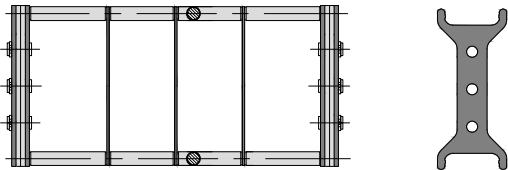
Çelik Dikey Separatör Uygulaması Steel Vertical Separator Application
